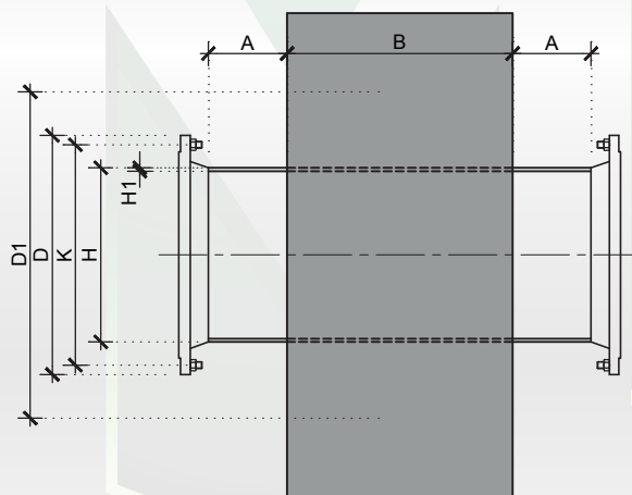
ΤΥΠΙΚΗ ΤΟΜΗ ΤΕΜΑΧΙΟΥ ΕΓΚΙΒΩΤΙΣΜΟΥ
