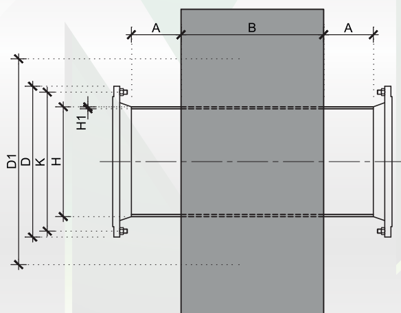
ΤΥΠΙΚΗ ΤΟΜΗ ΤΕΜΑΧΙΟΥ ΕΓΚΙΒΩΤΙΣΜΟΥ ΧΩΡΙΣ ΚΛΙΜΑΚΑ
